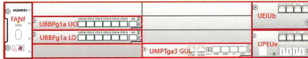
BBU5900-0-0
